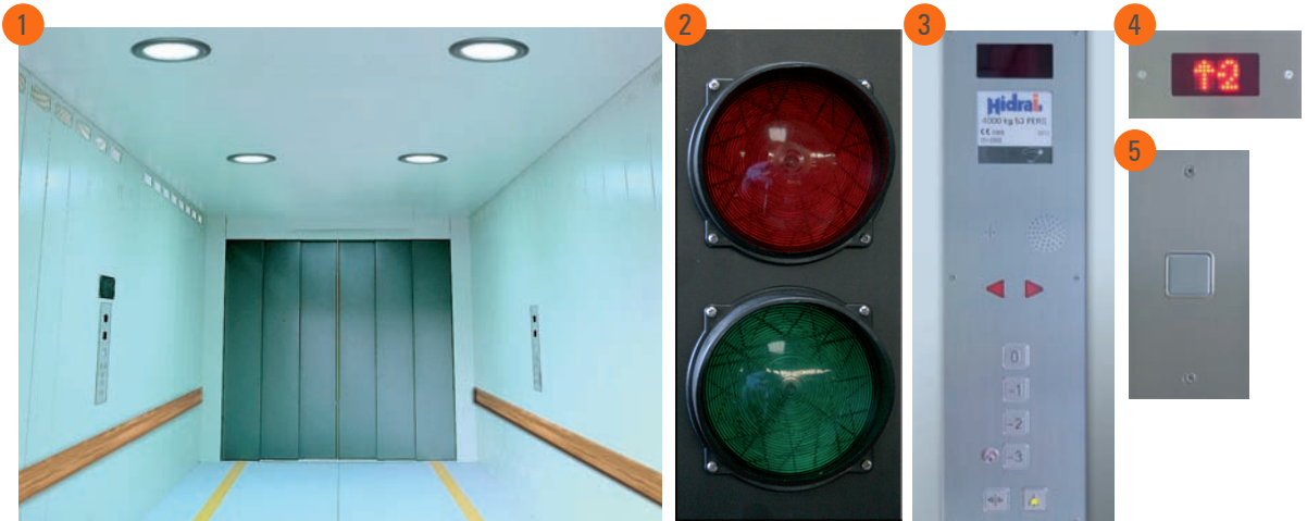
1. Cabina QHV. 2. Semáforo exterior. 3. Botonera de cabina con indicador de centrado de vehículos. 4. Indicador de posición en planta. 5. Botonera de planta.
