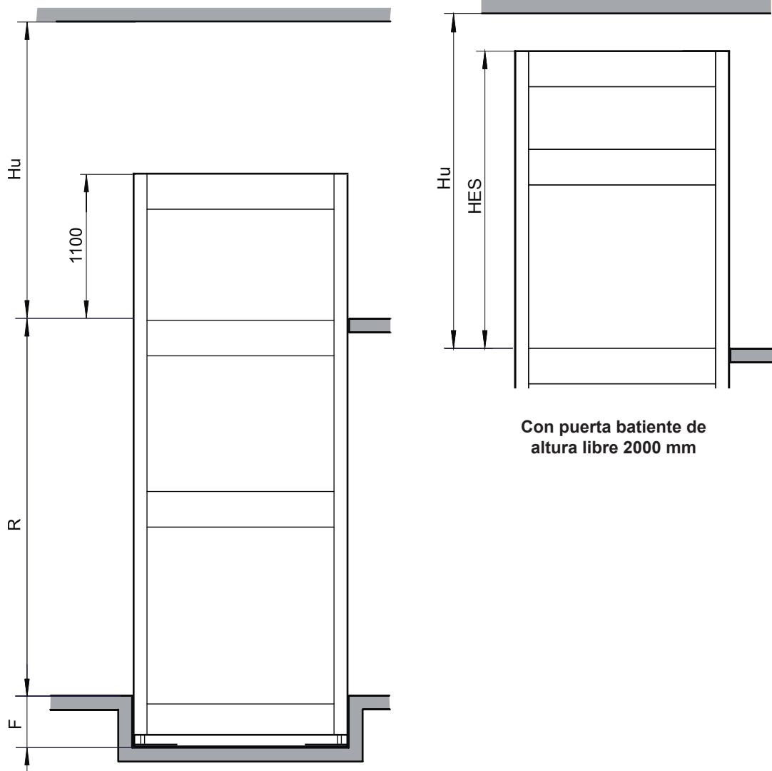
Con puerta batiente sin dintel de altura 1100 en el nivel superior
